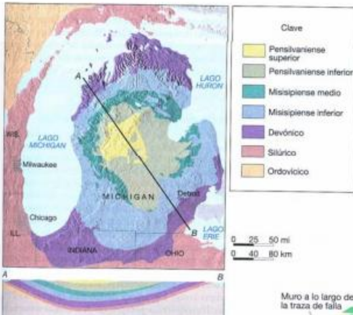
Figura 15.14 Geología del baso de la cuenca de Michigan. Obsérvese que las rocas más jóvenes están localizadas en el centro, mientras que los estratos más antiguos flanquean la estructura.
