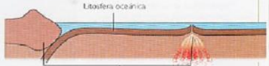
Placa oceánica
