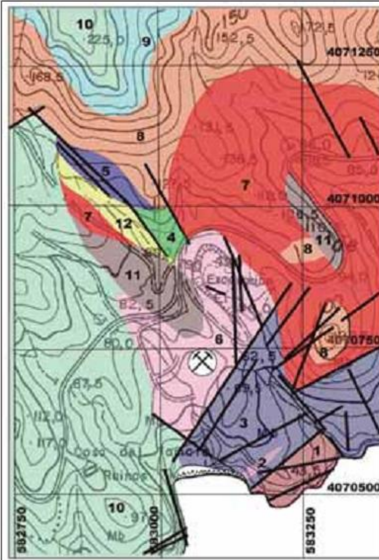
Figura 3. Ejemplo de mapa geológico realizado para un estudio geominero en Almería.
