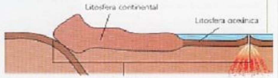
Placa mixta
