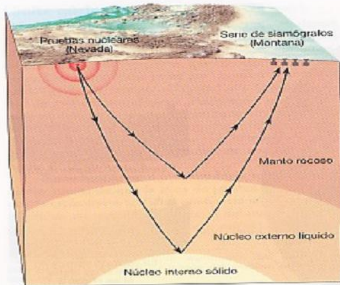
Figura 17.11 Se utilizaron los tiempos de desplazamiento de las ondas sísmicas generadas en pruebas nucleares para medir con exactitud la profundidad del núcleo interno. Una serie de sismógrafos localizados en Montana detectó los "ecos" que rebotaron desde el límite del núcleo interno.
