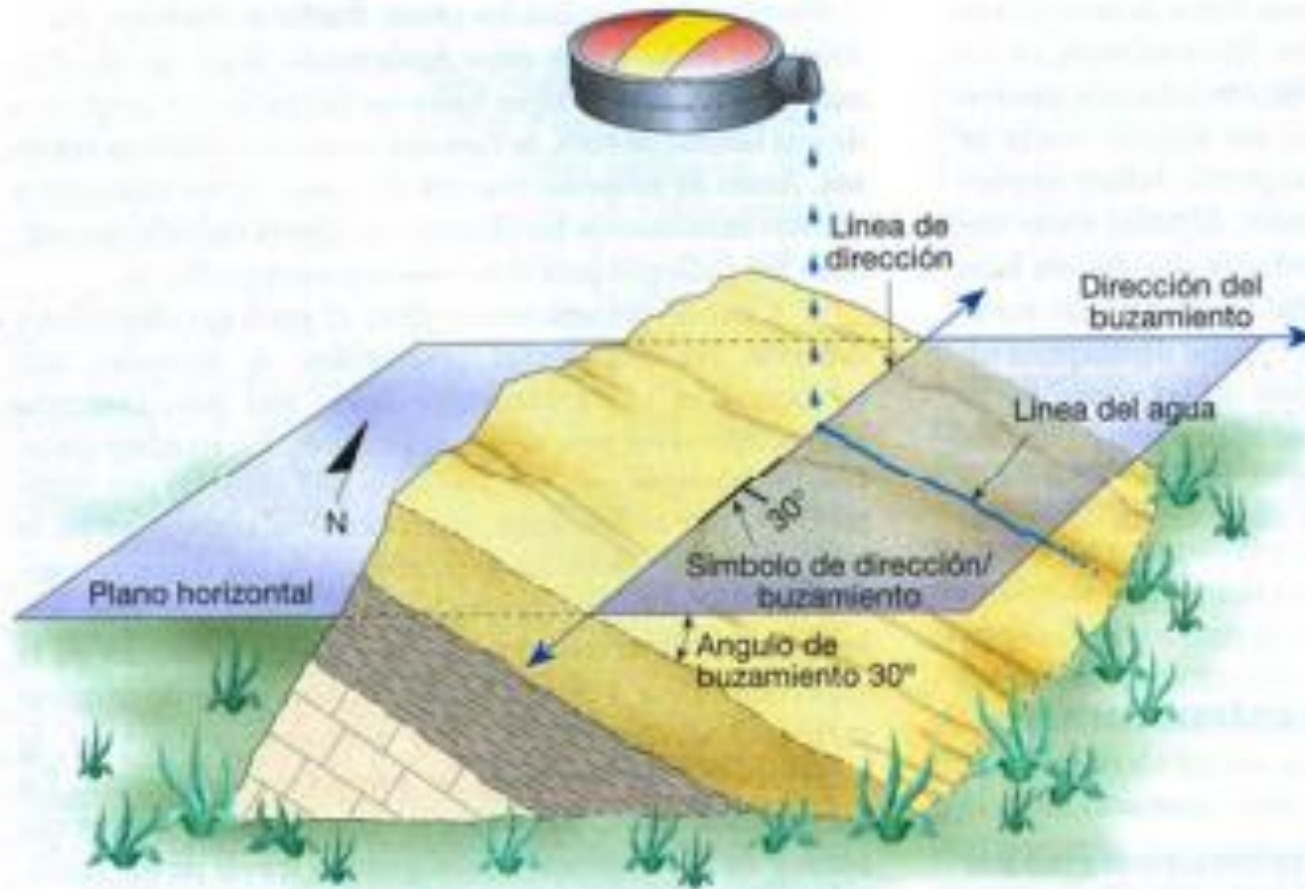
Figura 15.5 Dirección y buzamiento de un terreno rocoso.
